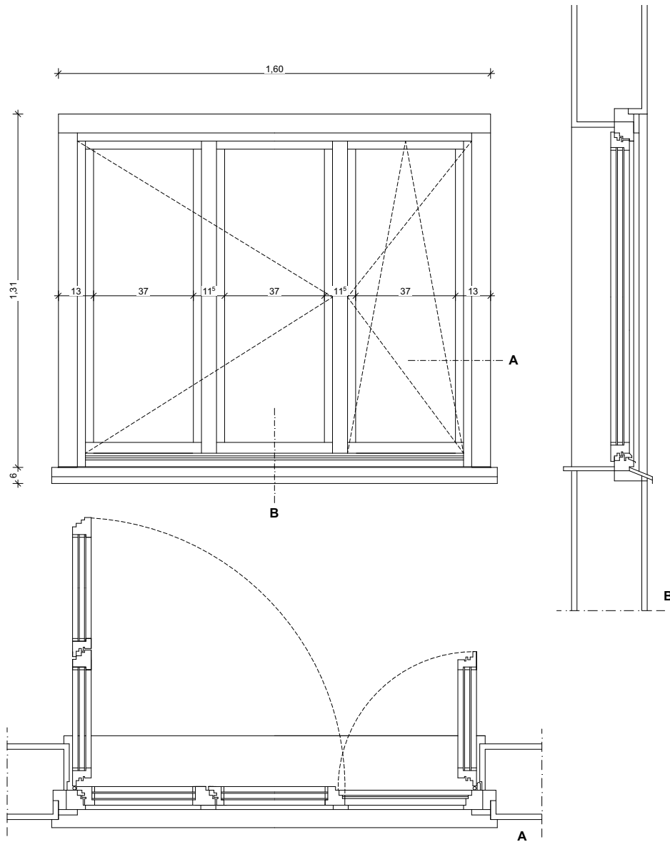
Ansicht, Horizontal- und Vertikalschnitt Dreiflügliges Fenster M 1:20
