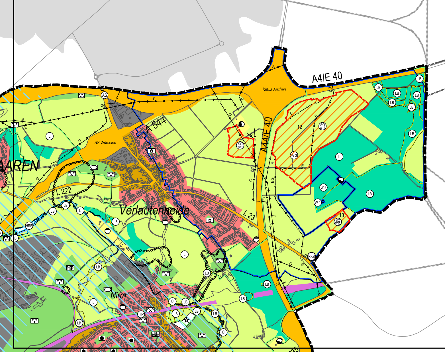
Teilausschnitt B
