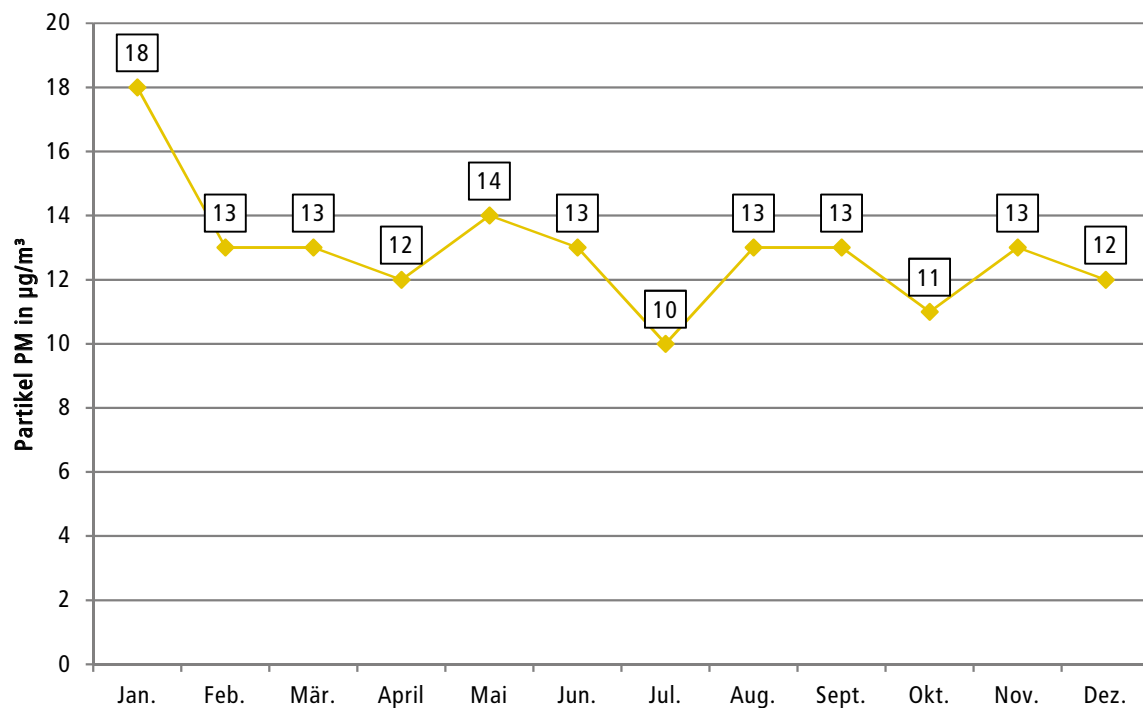
Abbildung 22: Feinstaub (PM 10 ) Aachen (in µg/m 3 Luft) im Jahr 2024; Messstation Aachen Burtscheid.
