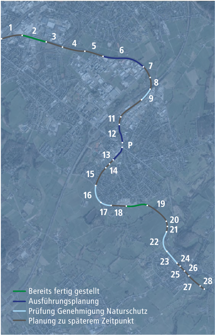
Abb.5: Bauabschnitte Vennbahnweg
